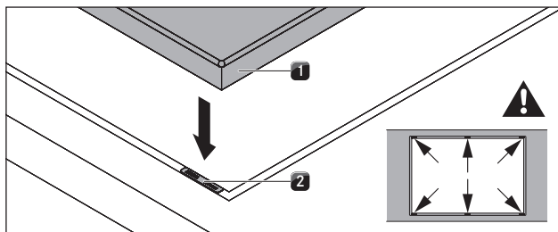
Afb. 6.21 Vulplaatjes invoegen
