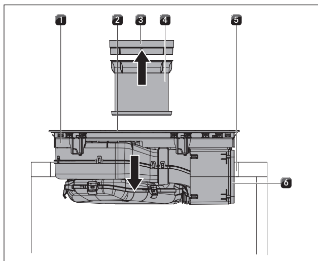
Afb. 6.33 Centrale plaatsing kookveld
