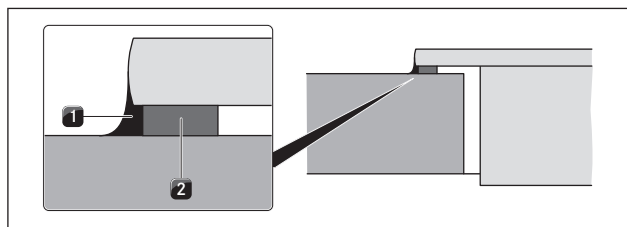
Afb. 6.29 Afdichtingsband bij opbouwmontage
