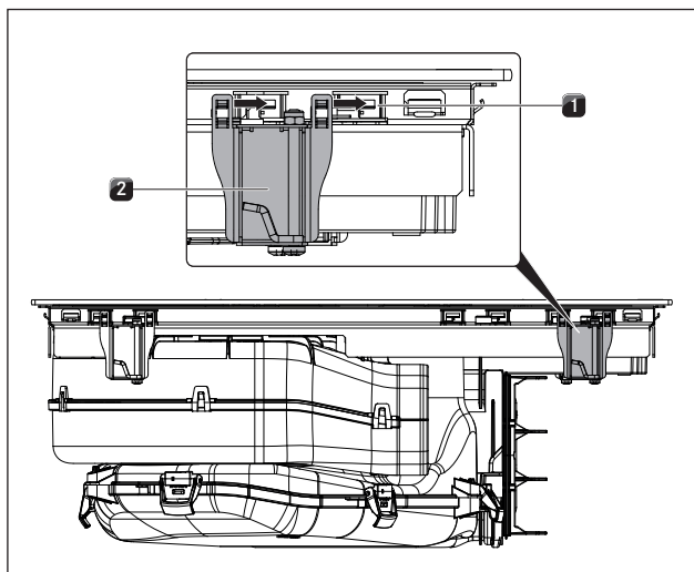
Afb. 6.19 Kookveld plaatsen
