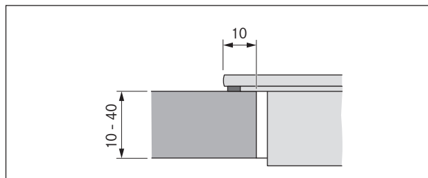
Afb. 6.11 Oplegmaat voor opbouwmontage
