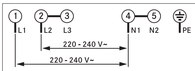
Afb. 6.45 Aansluitschema 2-fasig
