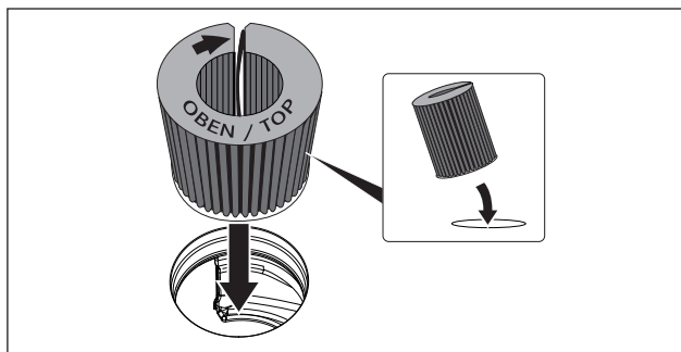
Afb. 6.40 Actieve-koolfilter in afzuigopening plaatsen
