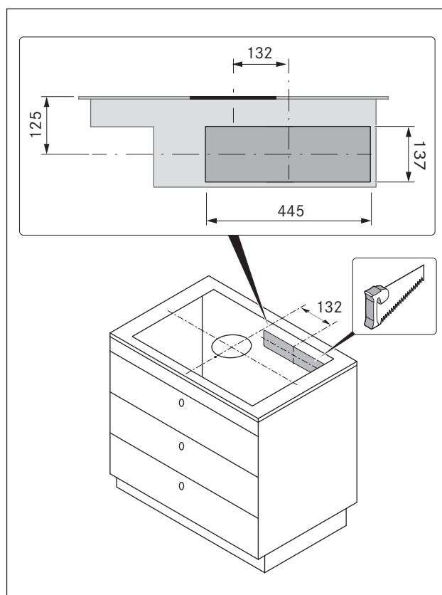
Afb. 6.27 Uitsparing van terugstroomopening
