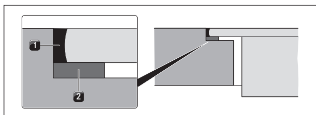
Afb. 6.30 Afdichtingsband bij vlainbouw
