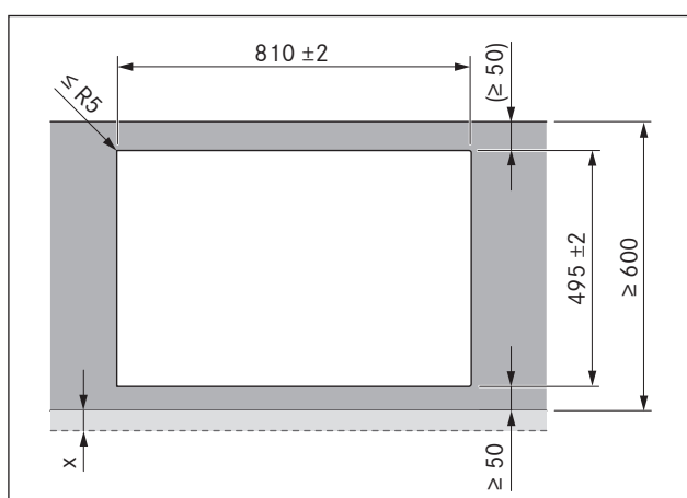
Afb. 6.10 Maten van de uitsparingen voor opbouwmontage
