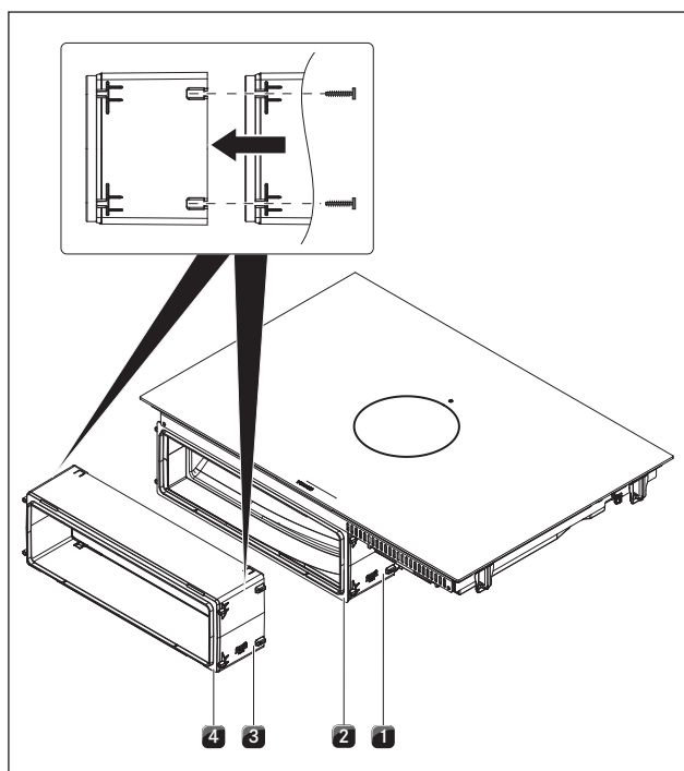
Afb. 6.32 Verlenging telescopisch kanaal.
