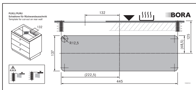
Afb. 6.28 Sjabloon voor achterwanduitsparing
