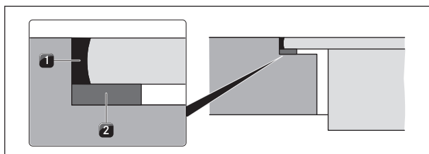
Afb. 6.18 Afdichtingsband bij vlakbouw
