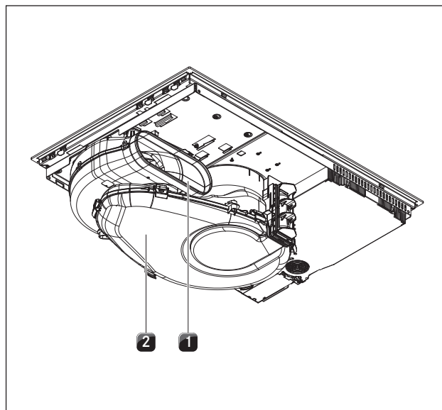
Afb. 5.2 Achteraanzicht PUXA, PURA
