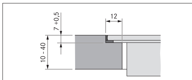
Afb. 6.13 Voegmaat voor vlakinbouw
