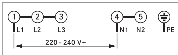
Afb. 6.46 Aansluitschema 1-fasig
