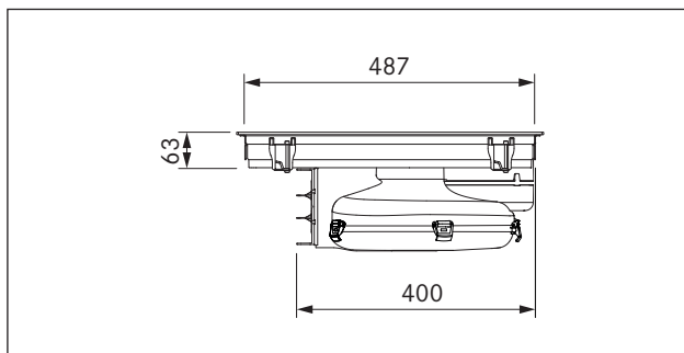
Afb. 3.3 PUXA toestelafmetingen zijaanzicht
