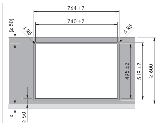
Afb. 6.12 Maten van de uitsparingen voor vlakinbouw
