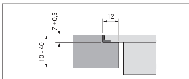
Afb. 6.9 Voegmaat voor vlakinbouw
