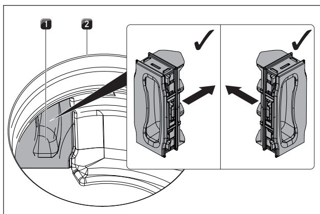
Afb. 8.11 Filtervervangingsklep plaatsen
