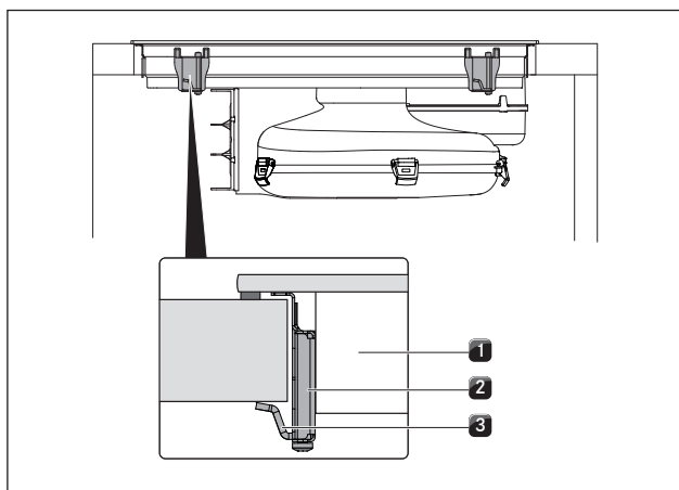
Afb. 6.23 Centrale bevestiging kookveld
