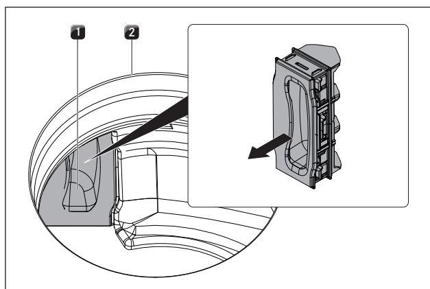
Afb. 8.5 Filtervervangingsklep verwijderen
