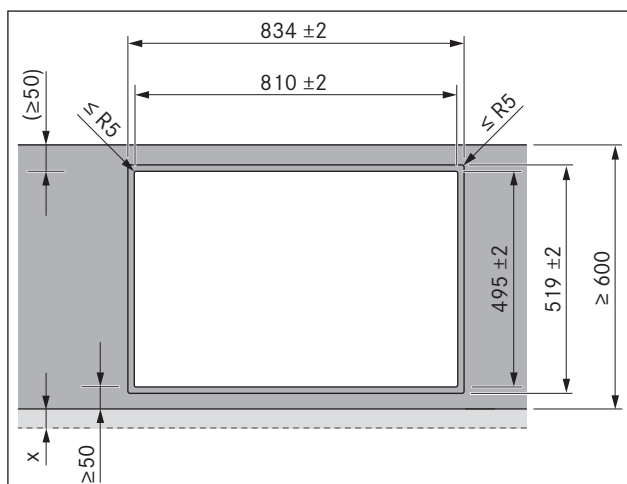
Afb. 6.8 Maten van de uitsparingen voor vlakinbouw
