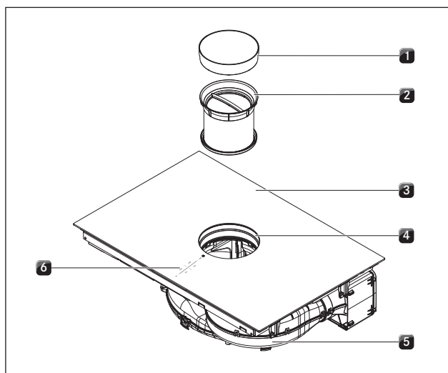
Afb. 5.1 Kookveld
