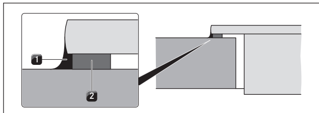
Afb. 6.17 Afdichtingsband bij opbouwmontage
