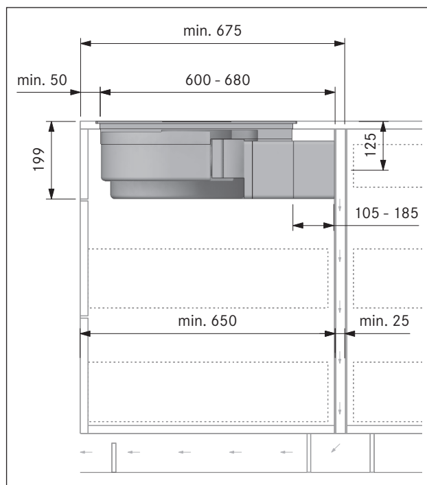
Afb. 6.26 Inbouwmaten bij recirculatie, werkbladdiepte vanaf 675 mm
