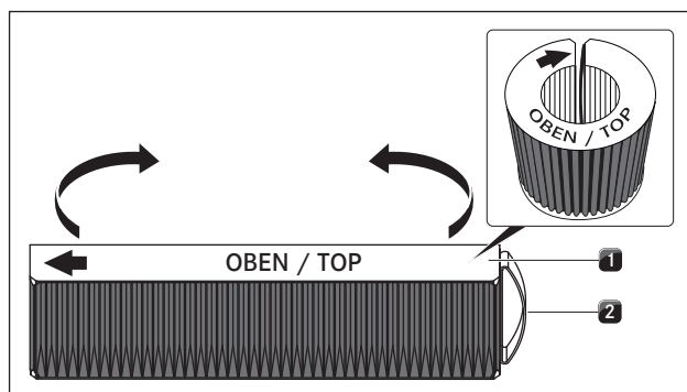
Afb. 8.8 Actieve-koolfilter
