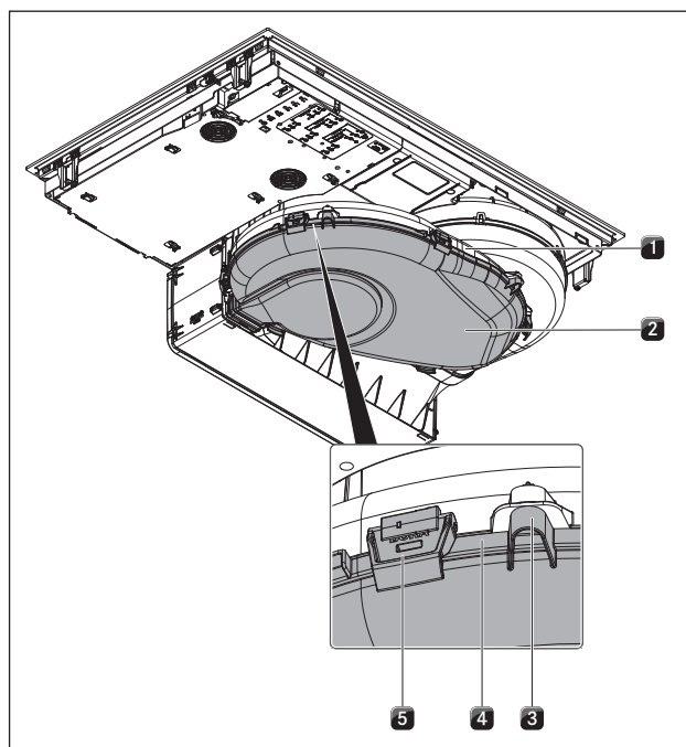
Afb. 8.4 Luchtgeleidingsbehuizing
