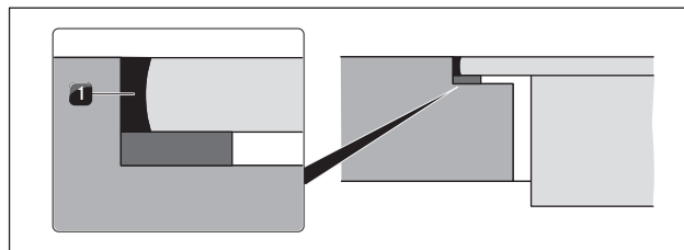
Afb. 6.53 Siliconenkit bij vlainbouw
