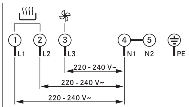
Afb. 6.44 Aansluitschema 3-fasig
