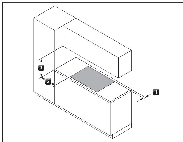
Afb. 6.3 voorgeschreven veiligheidsafstanden
