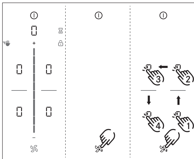
Afb. 6.48 Display dealer- en servicemenu oproepen
