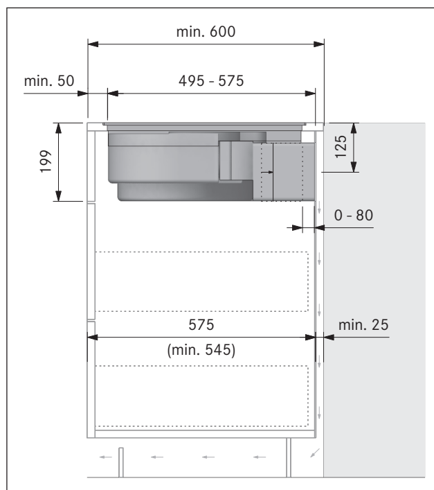
Afb. 6.25 Inbouwmaten bij recirculatie, werkbladdiepte 600 mm
